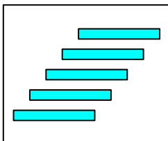
plot.shingle[bar.fill]
