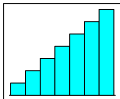
histogram[bar.fill]
