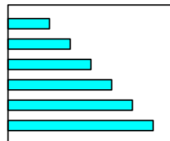
barchart[bar.fill]
